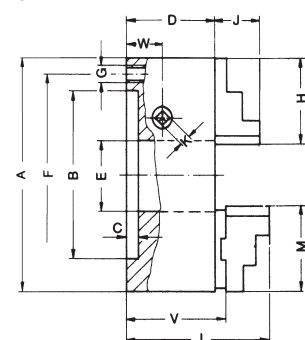
Cylindrical centre mount DIN 6350
