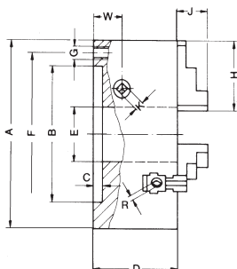
Cylindrical centre mount DIN 6351
